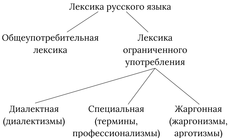
Рис. 5. Лексика с точки зрения сферы ее употребления
